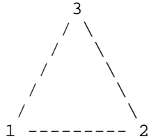
ESMF_MESHELEMENTTYPE_TRI
