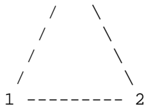
ESMF_MESHELEMENTTYPE_TRI
